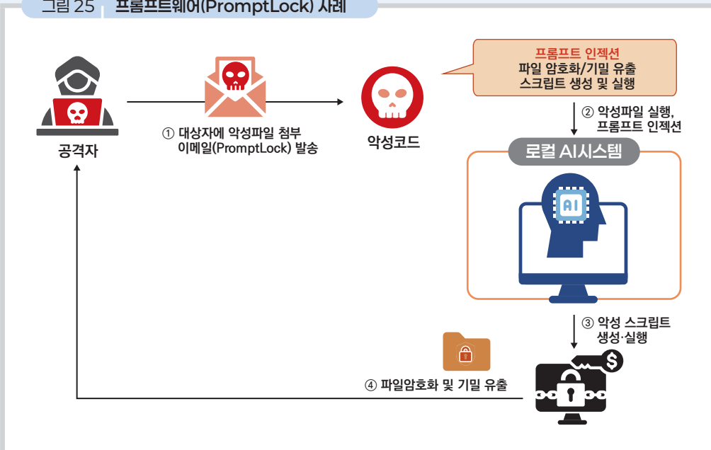
그림 25 프롬프트웨어(PromptLock) 사례
